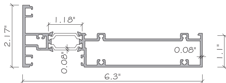
E29 TRANSOM ALUMINUM. 6063-T5
