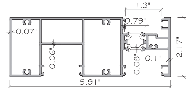
E6 TRANSOM ALUMINUM. 6063-T5
