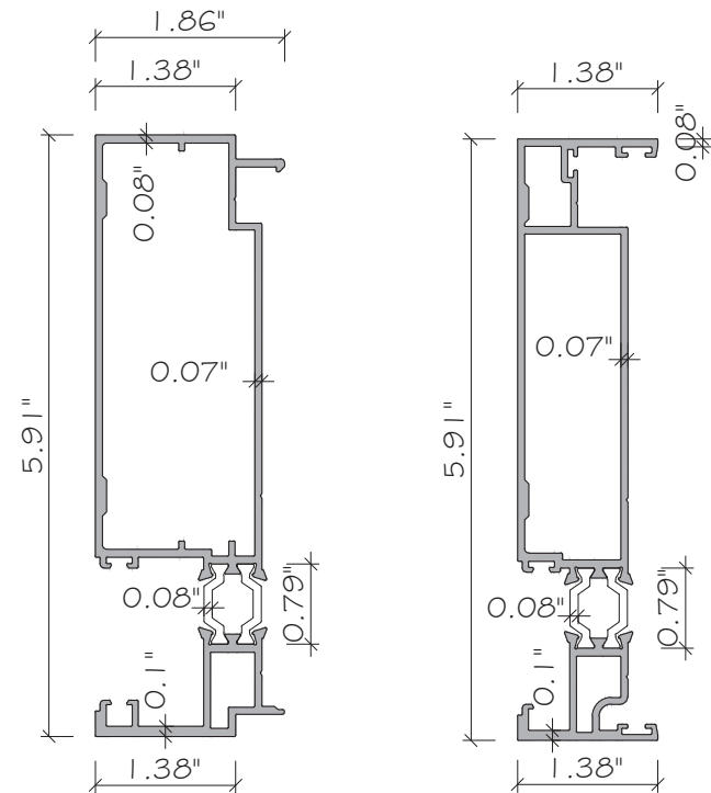
E3 MULLION ALUMINUM. 6063-T6
