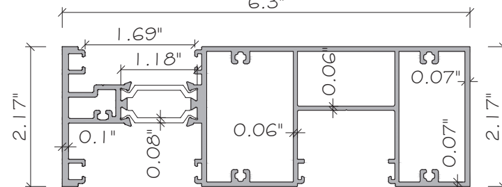
E30 TRANSOM ALUMINUM. 6063-T5
