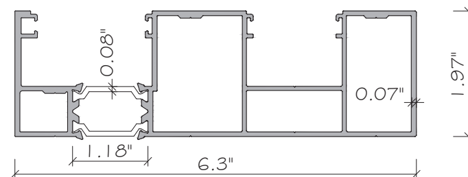
E26 FRAME JAMB ALUMINUM. 6063-T6
