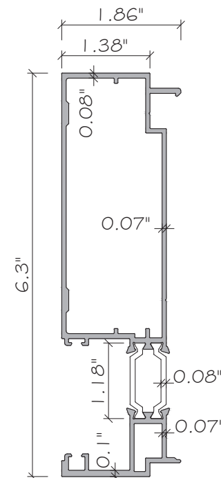
E27 MULLION ALUMINUM. 6063-T6
