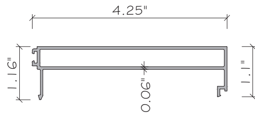
E7 GLASS BEAD ALUMINUM. 6063-T5
