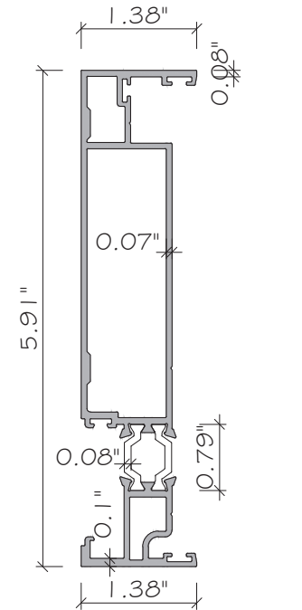
E4 MULLION ALUMINUM. 6063-T6
