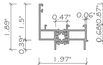
E12 FRAME FOR SASH ALUMINUM. 6063-T5
