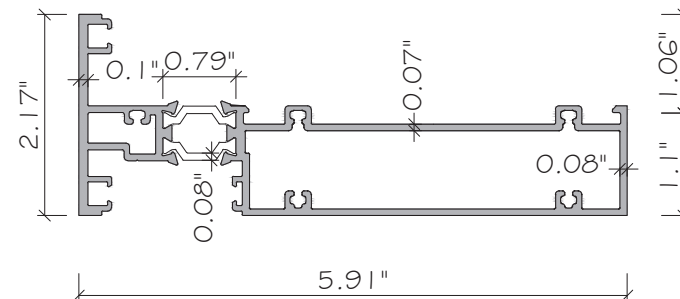
E5 TRANSOM ALUMINUM. 6063-T5
