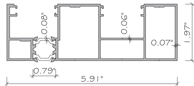
E2 FRAME JAMB ALUMINUM. 6063-T6
