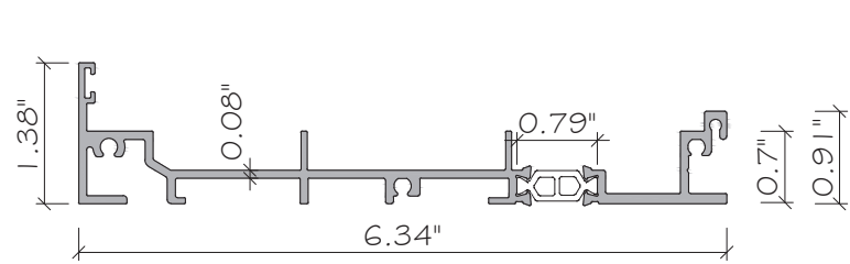
E1 SILL ALUMINUM. 6063-T5
