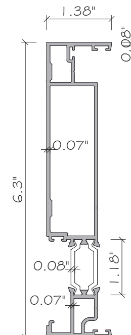
E28 MULLION ALUMINUM. 6063-T6
