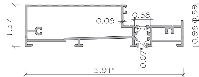
E20 DOOR SILL ALUMINUM. 6063-T5
